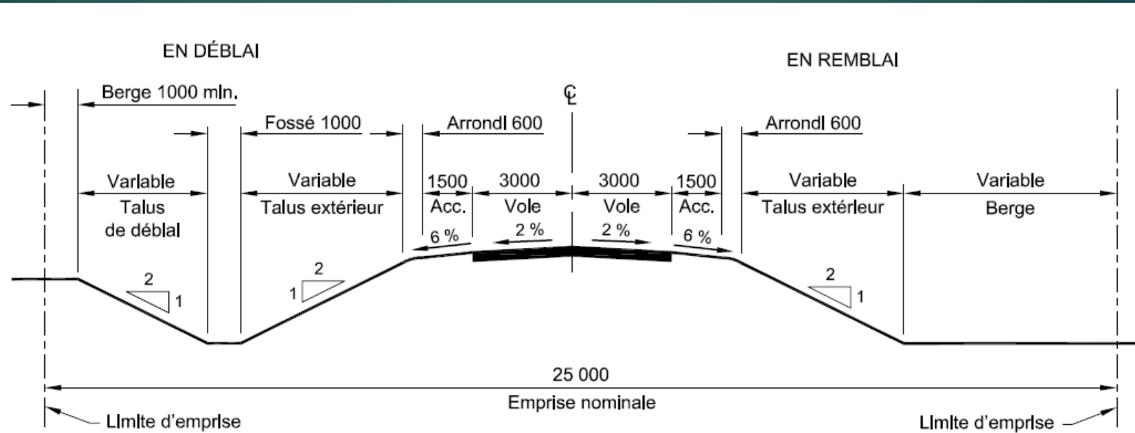
TYPE E : ROUTE RÉGIONALE – COLLECTRICE OU LOCALE
